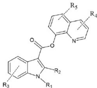
ESTRUTURA B12
